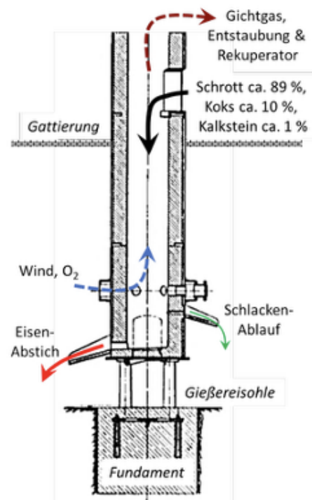
Prinzipskizze eines Kupolofens (vgl. 4 )
